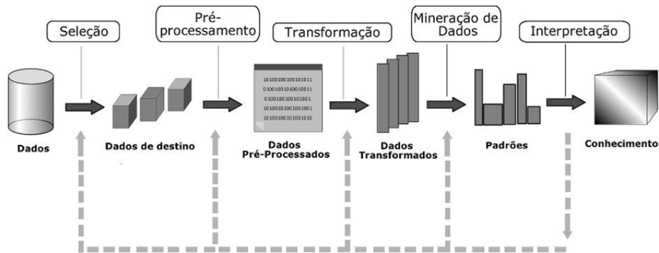
Figura 6 – Etapas do processo KDD.
