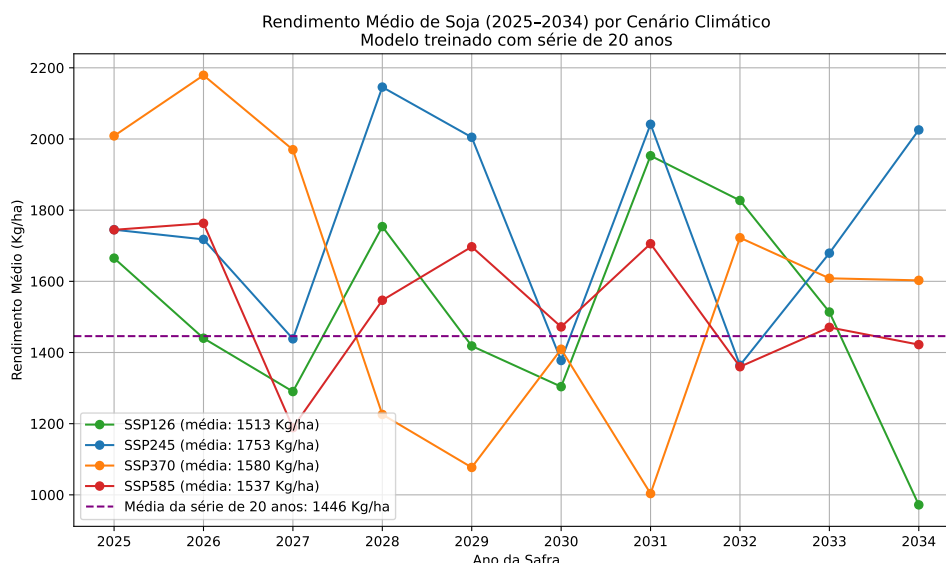
Figura 24 – Previsão Rendimento Médio da Soja com Série de 20 anos.
