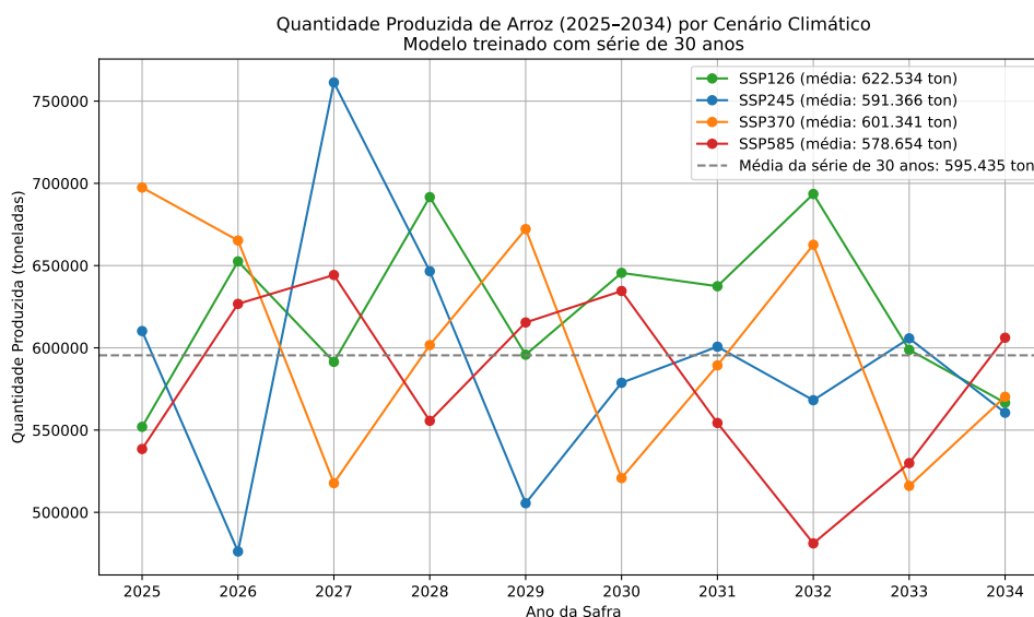
Figura 16 – Previsão Quantidade Produzida de Arroz com Série de 30 anos.
