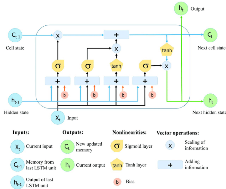
Figura 8 – Arquitetura de uma célula no modelo LSTM.
