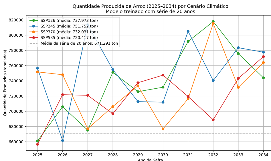
Figura 18 – Previsão Quantidade Produzida de Arroz com Série de 20 anos.
