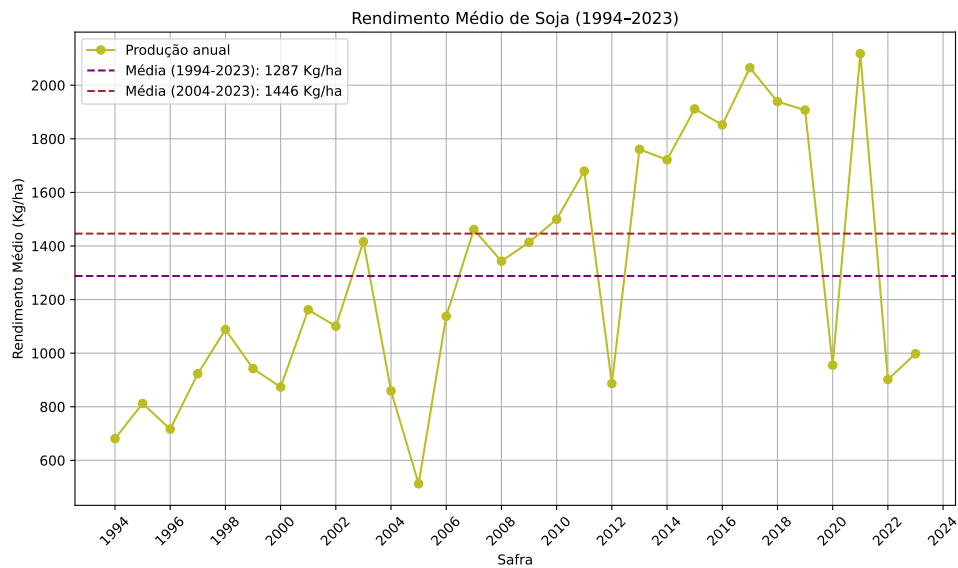
Figura 20 – Histórico de Rendimento Médio da Soja.
