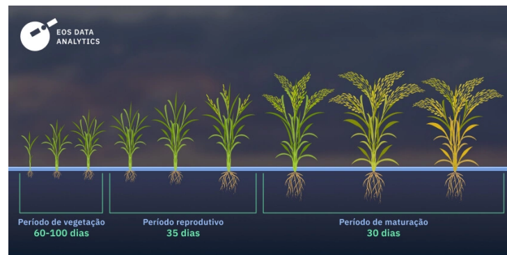
Figura 5 – Fenologia do Arroz.
