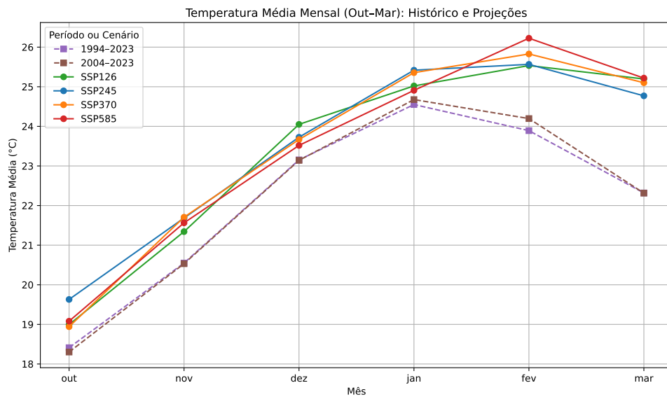
Figura 26 – Temperatura média nos meses de safra.
