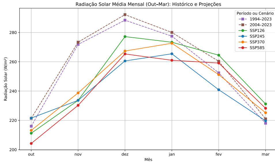
Figura 27 – Radiação solar nos meses de safra.
