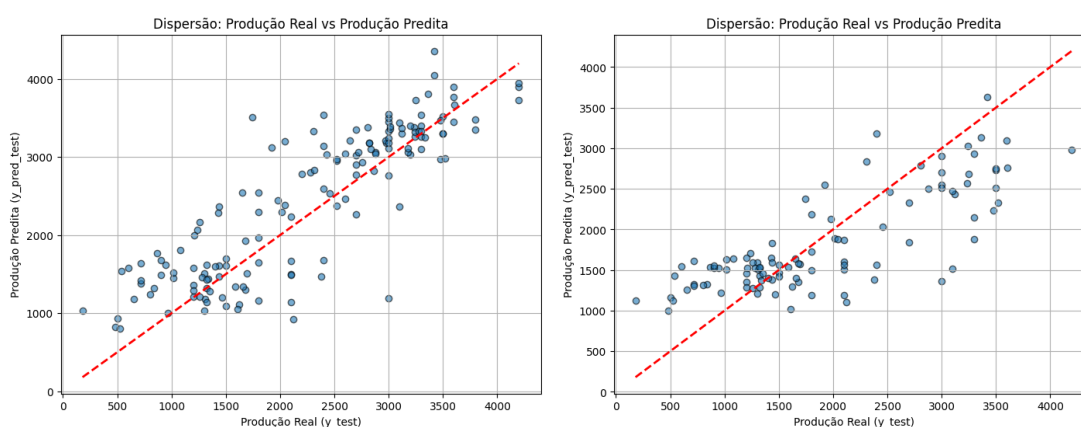
Figura 12 – Gráficos de Dispersão do conjunto de testes para Rendimento Médio de Soja nas Séries de 30 e 20 anos, respectivamente.
