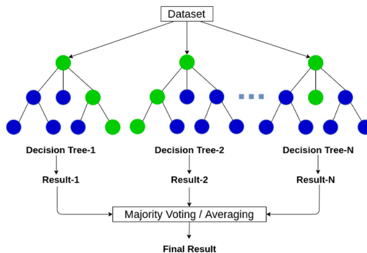
Figura 7 – Esquema do Random Forest.
