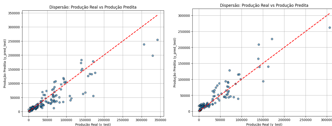
Figura 13 – Gráficos de Dispersão do conjunto de testes para Quantidade Produzida de Soja nas Séries de 30 (Modelo LSTM1) e 20 anos (Modelo LSTM2), respectivamente.
