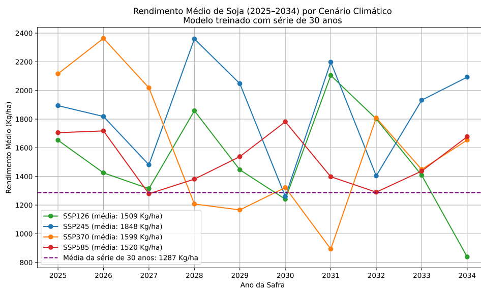
Figura 22 – Previsão Rendimento Médio da Soja com Série de 30 anos.
