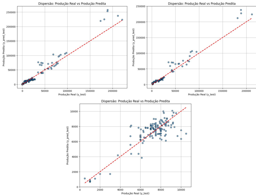
Figura 11 – Gráficos de Dispersão do conjunto de testes para Quantidade Produzida nas Séries de 30 e 20 anos e Rendimento Médio na Série de 20 anos, respectivamente.
