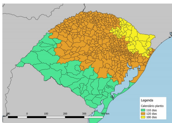
Figura 3 – Calendário do cultivo de soja no RS para a safra 2022/2023
