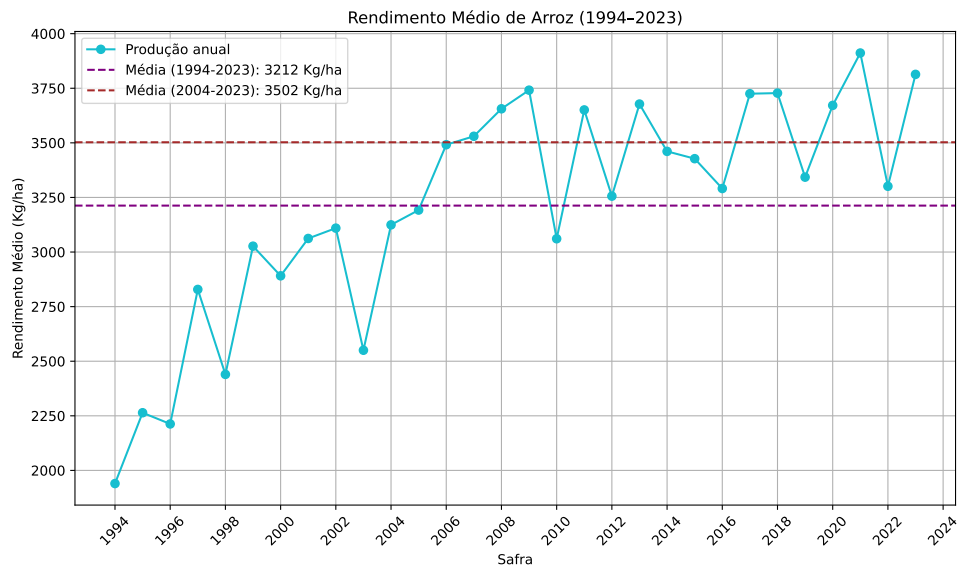
Figura 15 – Histórico de Rendimento Médio do Arroz.
