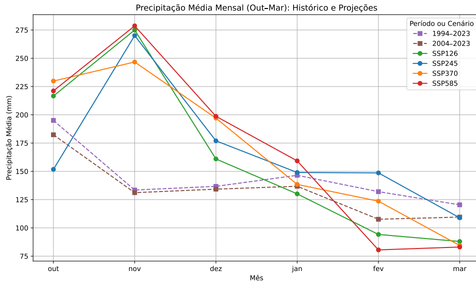
Figura 25 – Precipitação média nos meses de safra.
