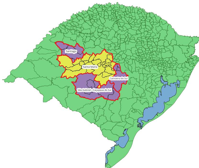
Figura 2 – Regiões Geográficas Imediatas contidas na Região Intermediária de SM
