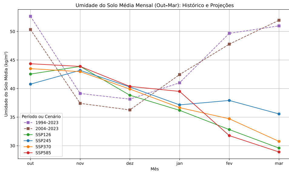
Figura 28 – Umidade do solo nos meses de safra.
