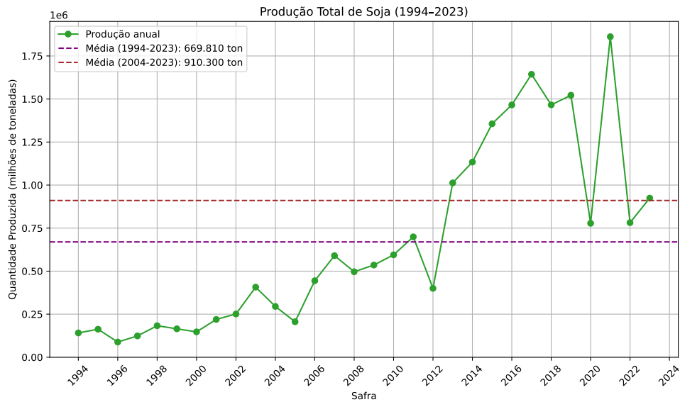
Figura 19 – Histórico de Quantidade Produzida de Soja.
