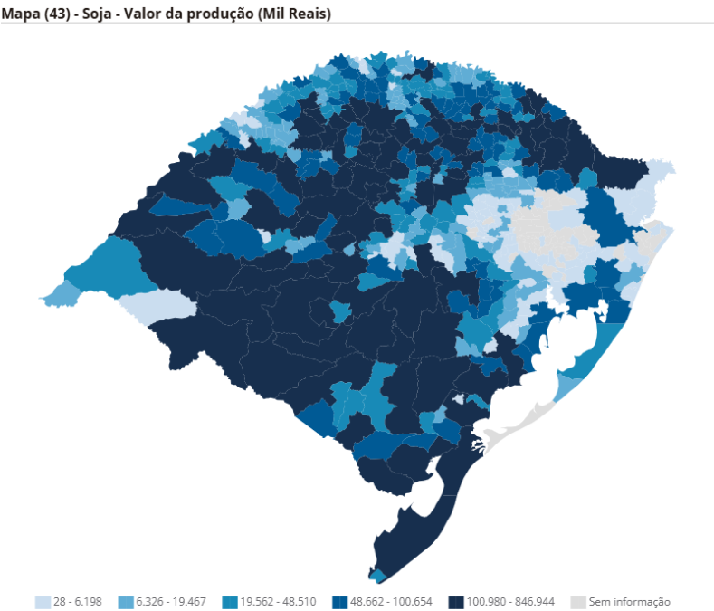
Figura 10 – Produção de Soja no RS em 2023.
