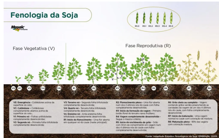
Figura 4 – Fenologia da Soja.
