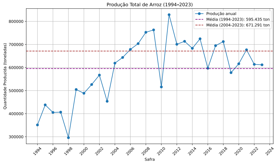
Figura 14 – Histórico de Quantidade Produzida de Arroz.
